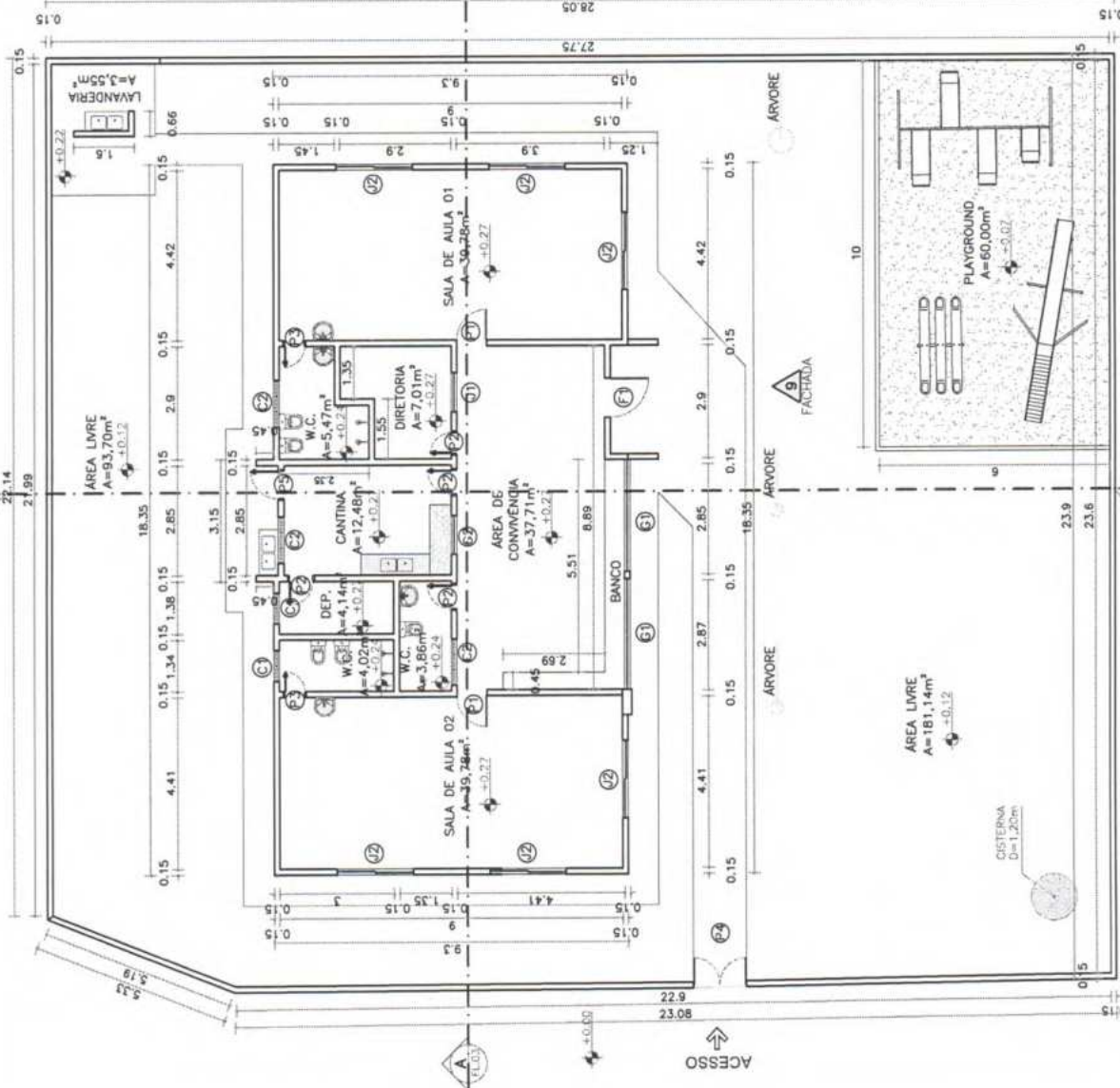
1 PLANTA BAIXA PROPOSTA ESC. 1:125
