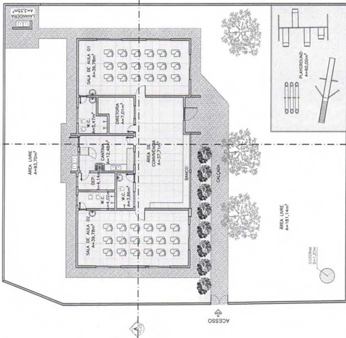
1 PLANTA LAYOUT PROPOSTA ESC. 1:125
