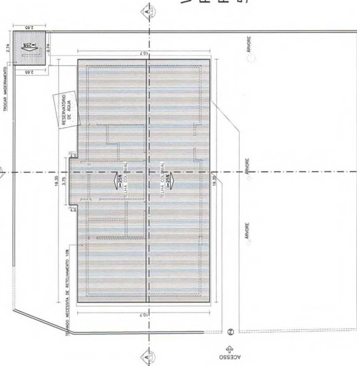
1 PLANTA DE COBERTA ATUAL ESC. 1:125
