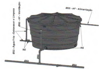
ISOM. CAIXA D'ÁGUA
