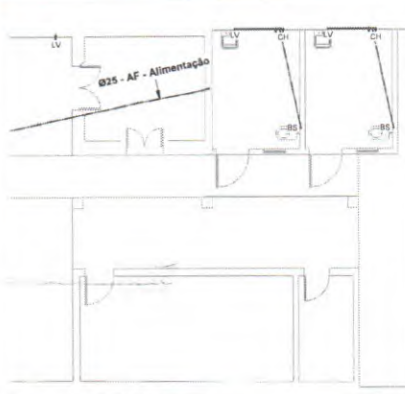
PLANTA - ÁGUA FRIA 1 : 100
