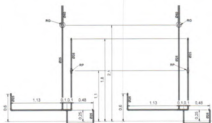
CORTE W.C.s 1 : 25
