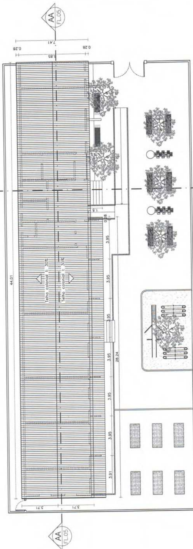
PLANTA DE COBERTA – PROPOSTA ESC. 1:150
